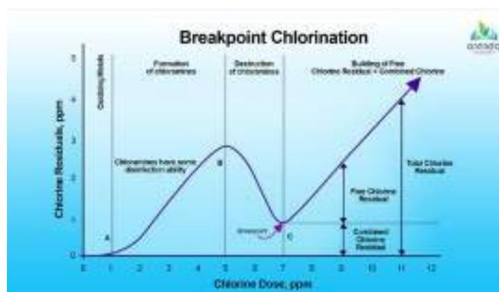
Figura 4. Fases de la demanda de cloro en solución acuosa y establecimiento del breakpoint
