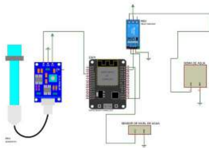
Figura 6. Diagrama de conexiones Fuente: Autores
