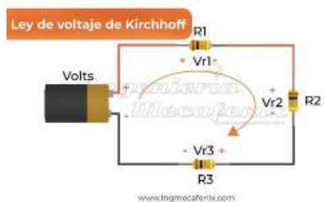
Figura 2. Circuito de ejemplo para verificar las leyes de Kirchhoff Fuente: [7]
